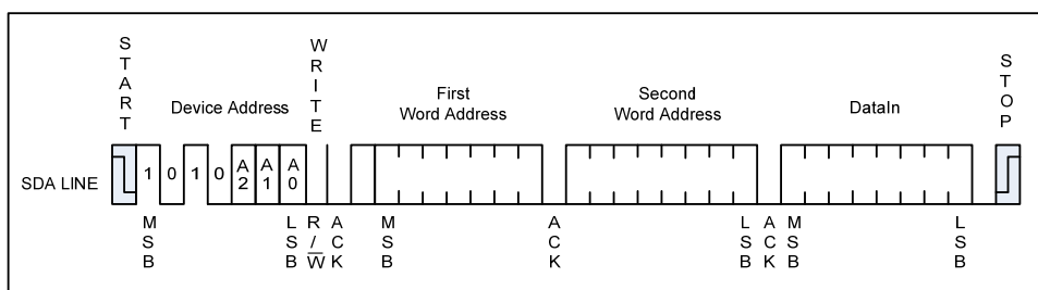
Figure6 Byte Write
