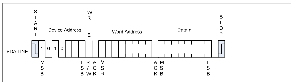
Figure5 Byte Write
