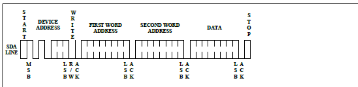
Figure4 Byte Write
