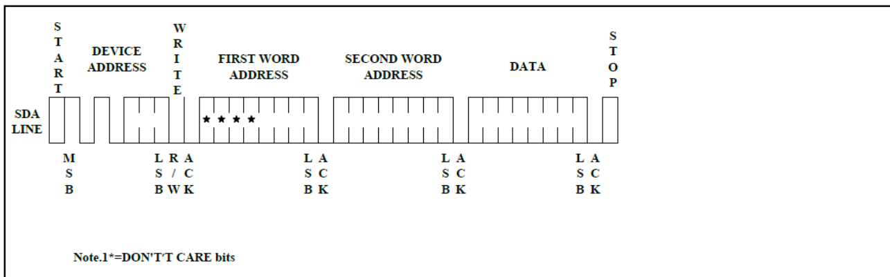
Figure4 Byte Write
