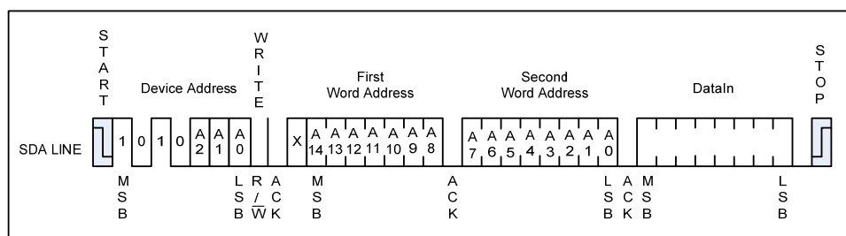
Figure9 Byte Write
